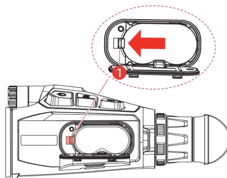
Gambar 2-4 Lepas Baterai
